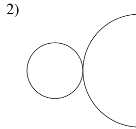
cone
